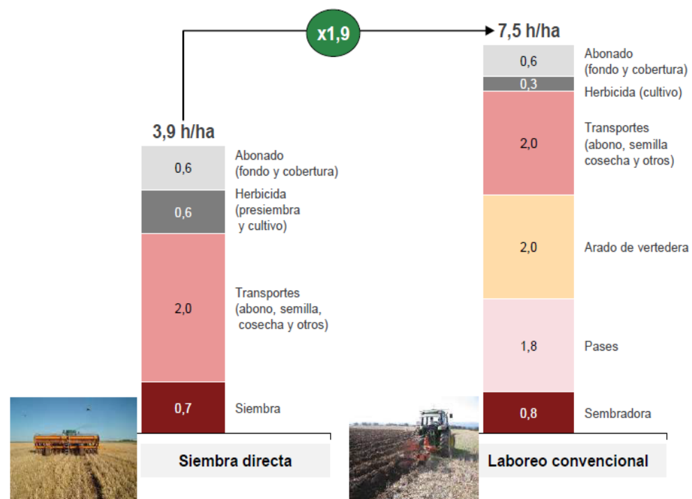
Comparativa de tiempos de trabajo en labores mecanizadas en Agricultura de Conservación frente a agricultura convencional (h/ha)
